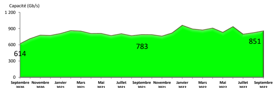
Evolution mensuelle de la capacité consommée
